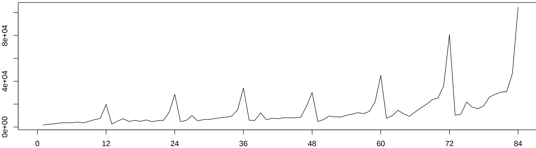
Raw Data Z
